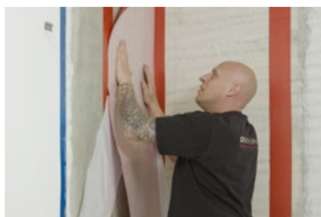
4. Dichtbahnen anbringen
