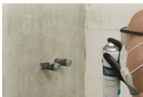
2. Primerspray auftragen
